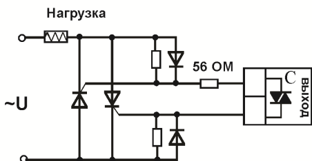
Подключение внешних тиристоров
