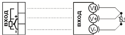
Рисунок 5 - Схема подключения термометра сопротивления к входу прибора
