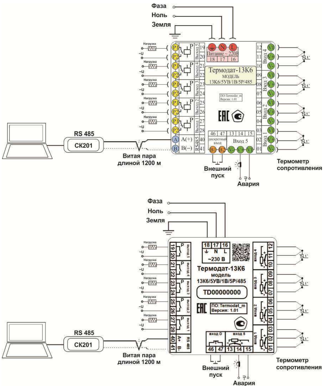
Рисунок 11 – Схема подключения прибора по 5 каналам
