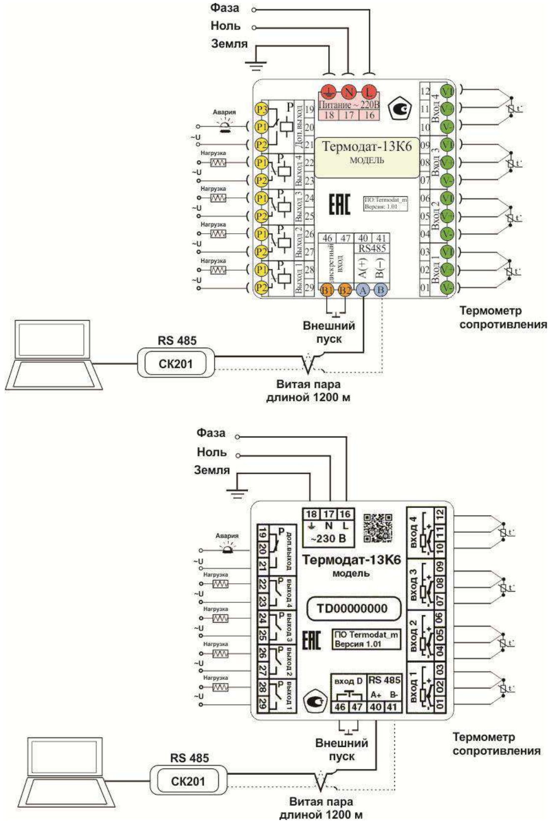
Рисунок 10 – Схема подключения прибора
