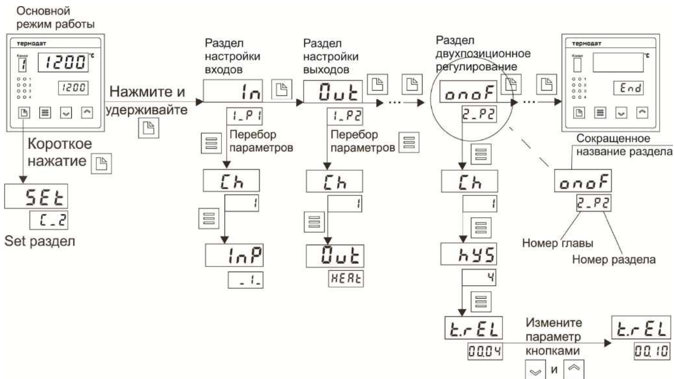
Рисунок 3 – Схема меню
