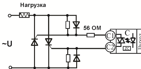
Подключение внешних тиристоров
