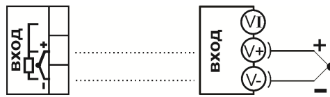
Рисунок 4 - Схема подключения термопары к входу прибора.
