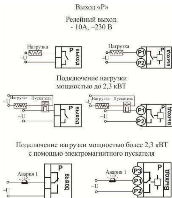
Рисунок 7 – Схемы подключения релейных выходов
